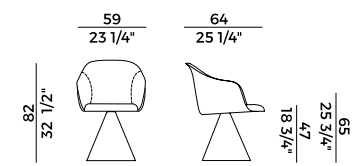
918/PGCI poltroncina base cono girevole \ cone base swivel armchair
