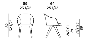
918/PI poltroncina \ armchair
