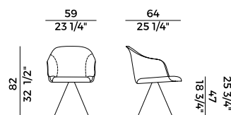
918/PGC poltroncina base cono girevole \ cone base swivel armchair
