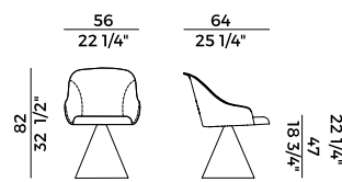
918/GCI sedia base cono girevole \ cone base swivel chair
