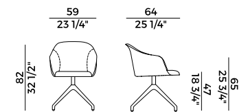
918/PGI poltroncina girevole \ swivel armchair
