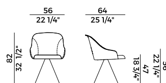
918/GCI sedia base cono girevole \ cone base swivel chair
