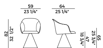
918/PGCI poltroncina base cono girevole \ cone base swivel armchair
